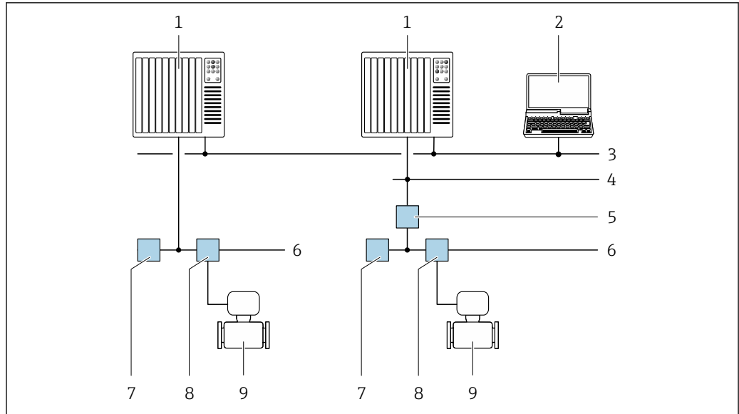
图 33 通过基金会现场总线(FF)网络进行远程操作
