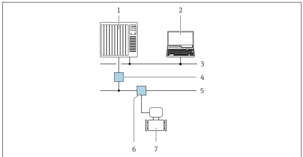
32 通过 PROFIBUS PA 网络进行远程操作
