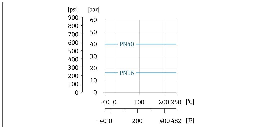
图 20 连接法兰的材质：铸钢 CX2MW，类似 Alloy C22/2.4602 合金
