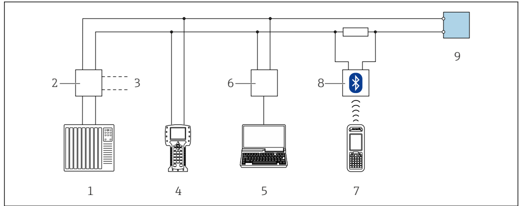
31 通过 HART 通信进行远程操作 (无源)
