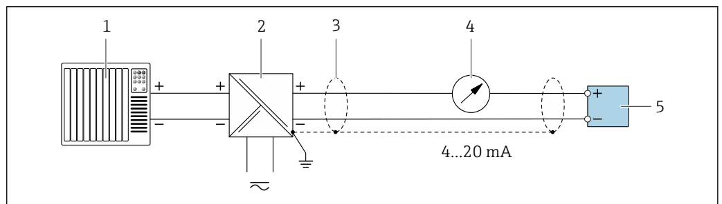
图 6 4...20 mA HART 无源电流输出的连接实例
