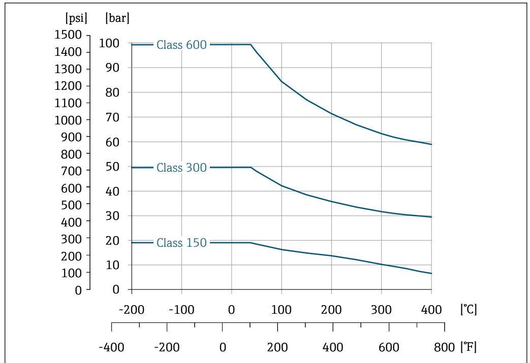
21 连接法兰的材质: 不锈钢 1.4404/F316/F316L, 多种材料认证
