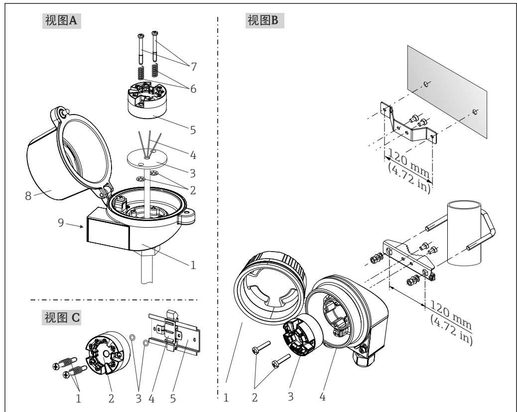
图 3 模块化变送器的安装示意图（三种安装方式）
