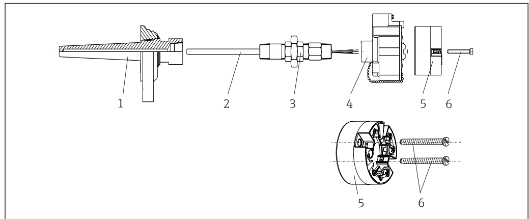
图 5 安装模块化变送器
