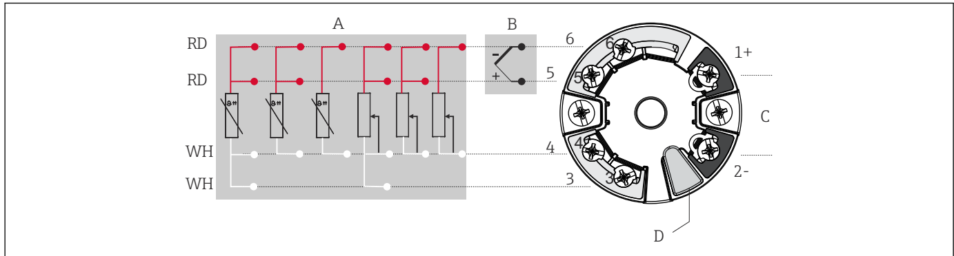
图 9 模块化变送器的接线端子分配
