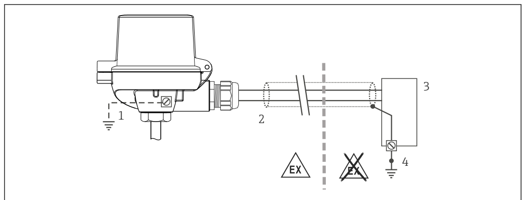
图 13 HART®通信电缆的单端屏蔽和接地连接
