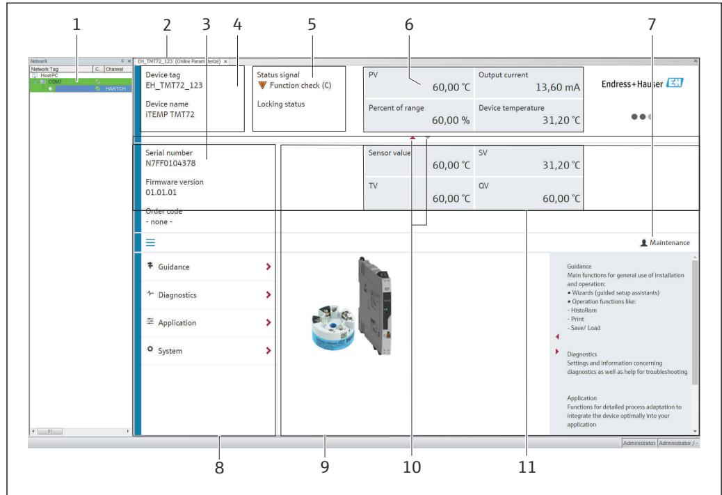
图 19 FieldCare 用户界面，显示设备信息
