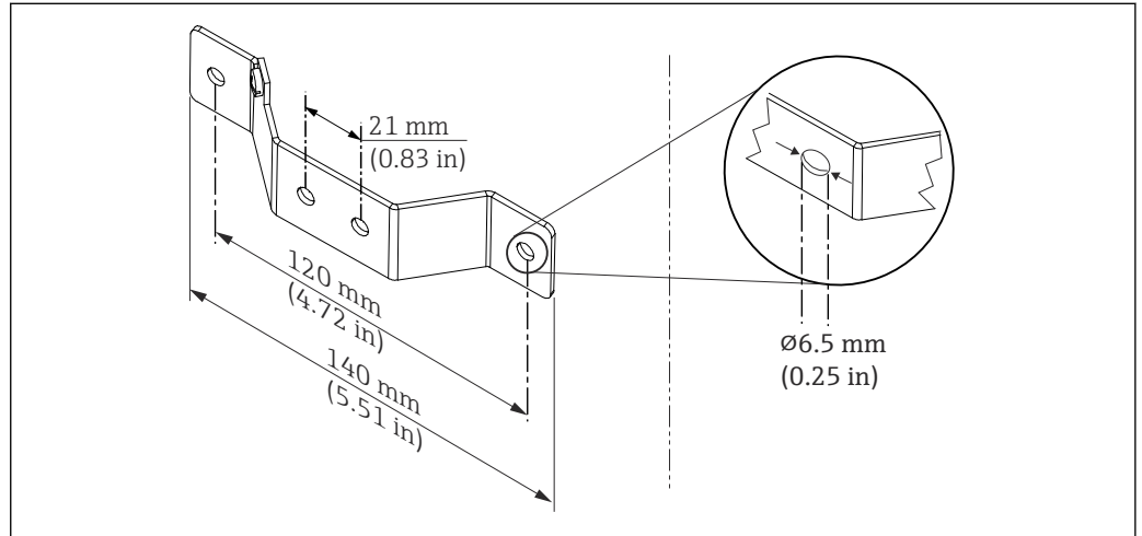
图 4 墙装架的外形尺寸（整套墙装套件可以作为附件订购）
