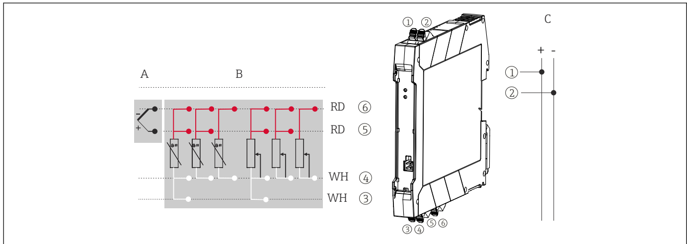
图 10 DIN 导轨型变送器的接线端子分配示意图
