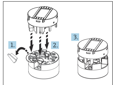
图 16 将显示单元安装在变送器上
