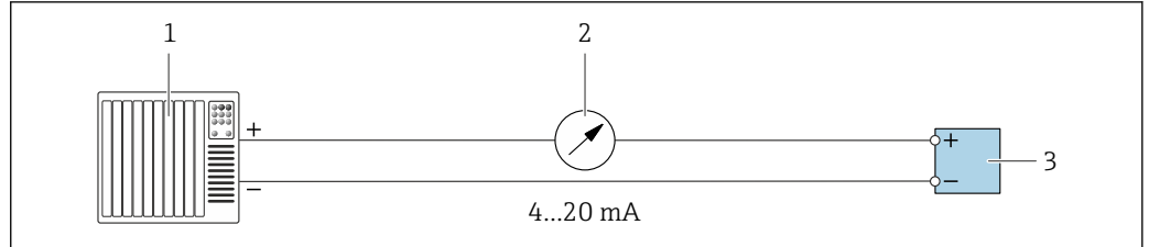
图 23 4...20 mA 有源电流输出的连接实例
