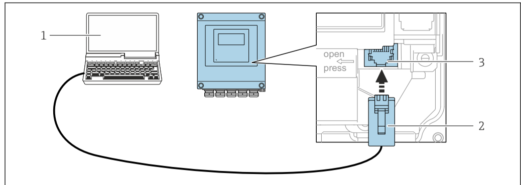
图 36 通过服务接口(CDI-RJ45)操作
