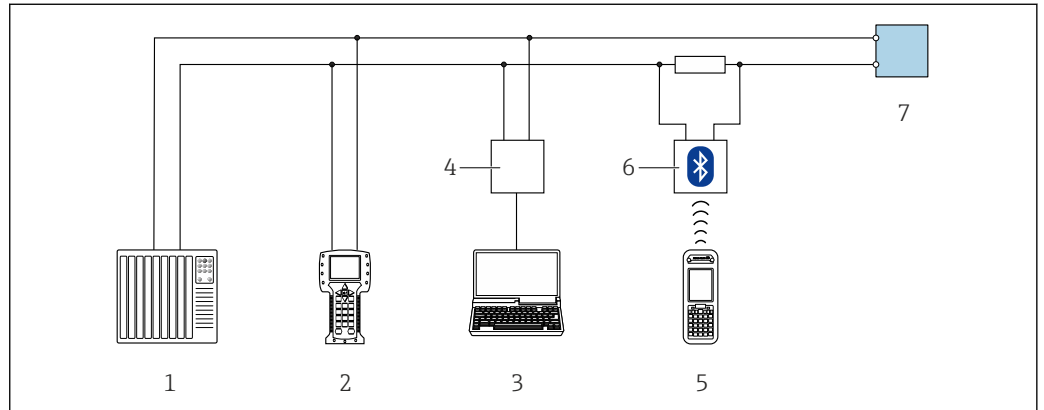
图 34 通过 HART 通信进行远程操作(有源信号)
