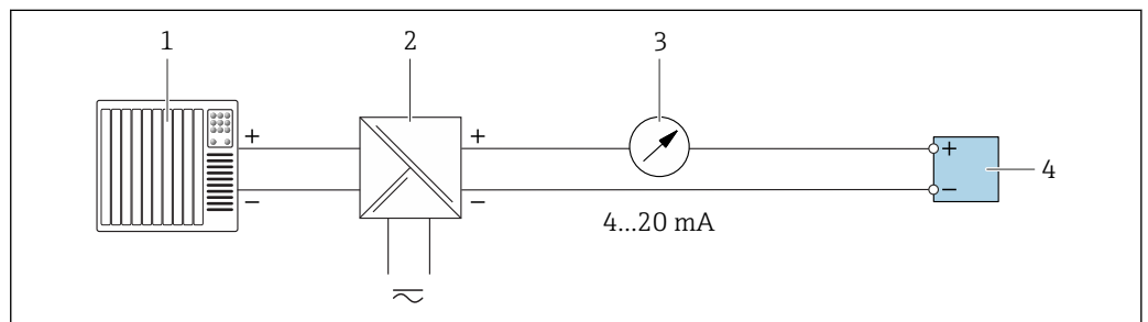
图 24 4...20 mA 无源电流输出的连接实例
