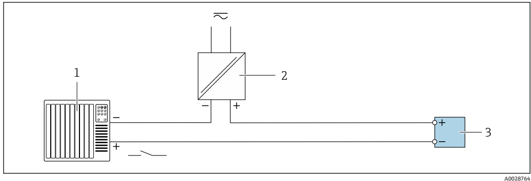
图 31 状态输入的连接实例
