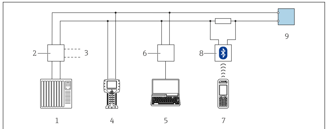
图 35 通过 HART 通信进行远程操作(无源信号)
