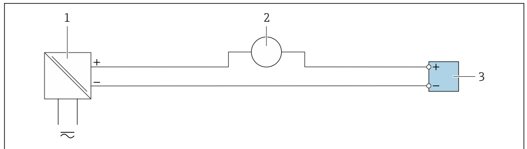
图 30 4...20 mA 电流输入的连接实例
