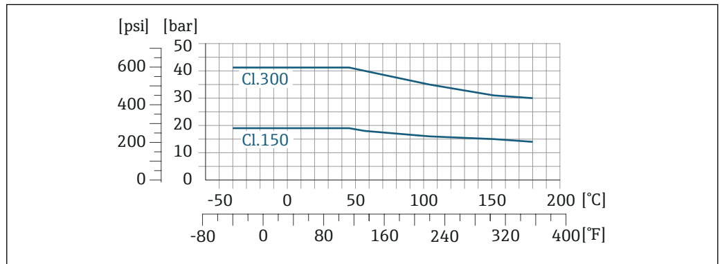
图 45 法兰材质: 1.4404/F316L/F316
