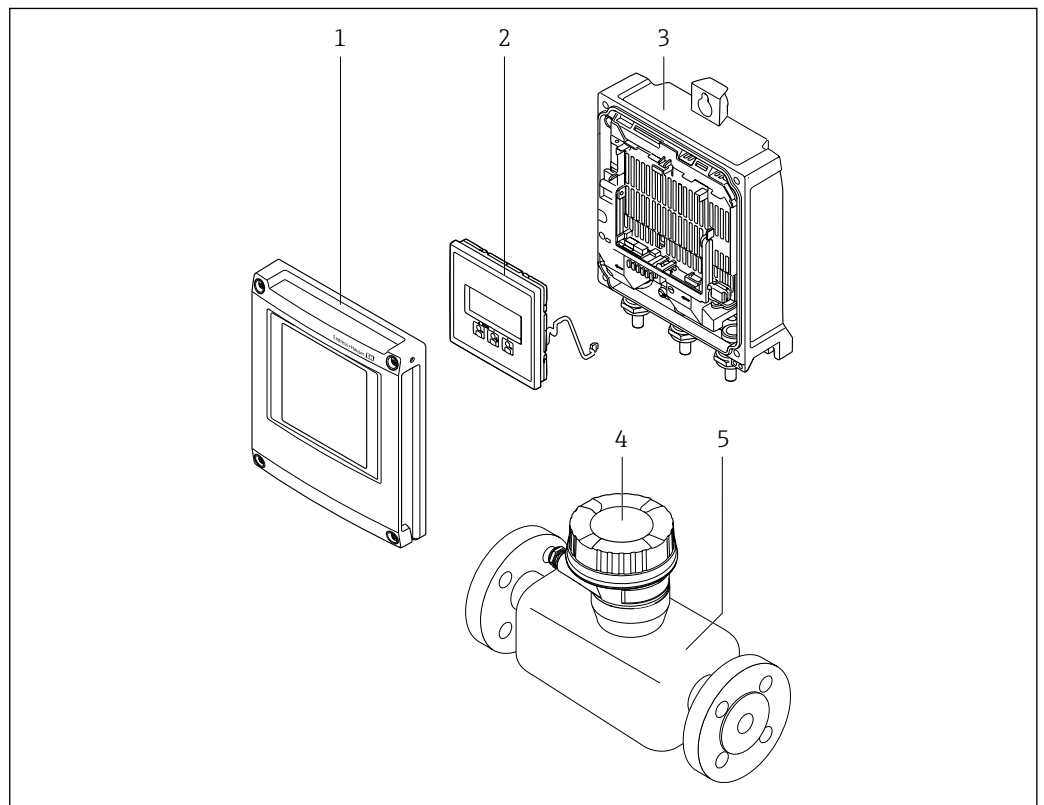
图 1 仪表主要组成部件
