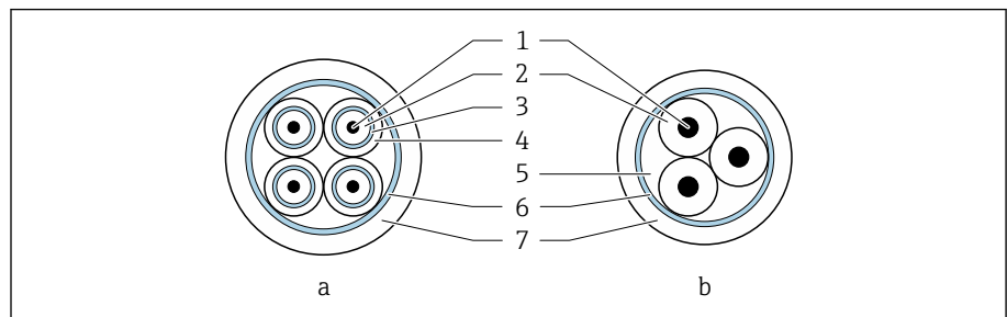
图 9 电缆截面图
