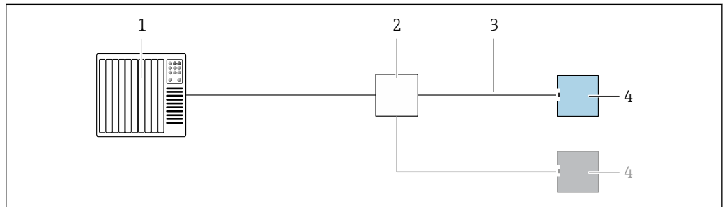
4 接线示例: 具有 Ethernet-APL 功能的 PROFINET
